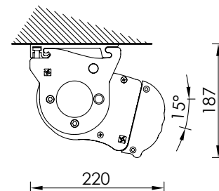
Montaggio a soffitto 15° Ceiling installation 15°
