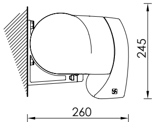
Dimensioni massime - Maxi dimensions
